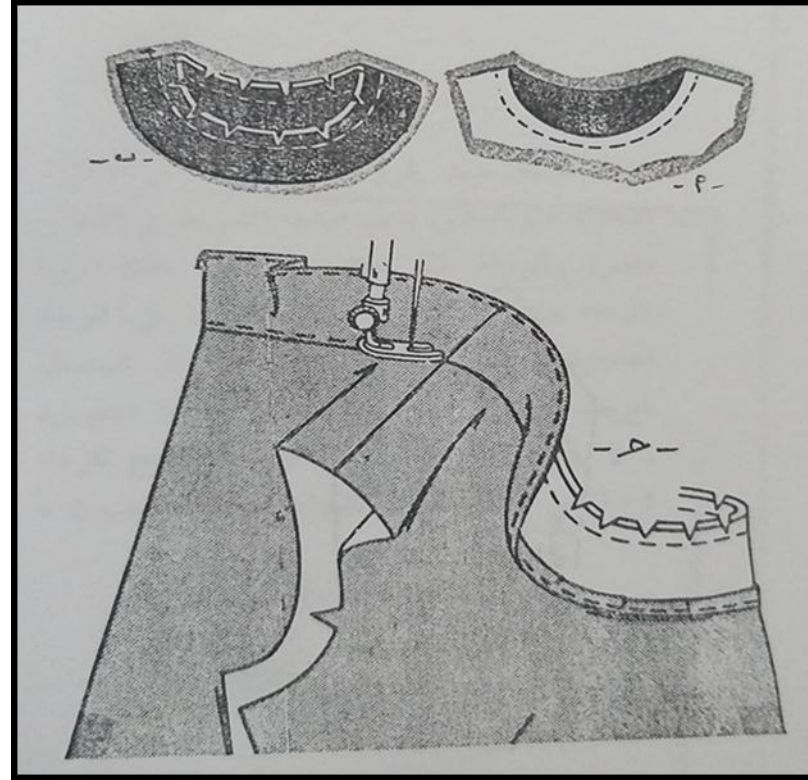
شكل ( ٣٦ ) اعداد تقوية الرقبة المستديرة
