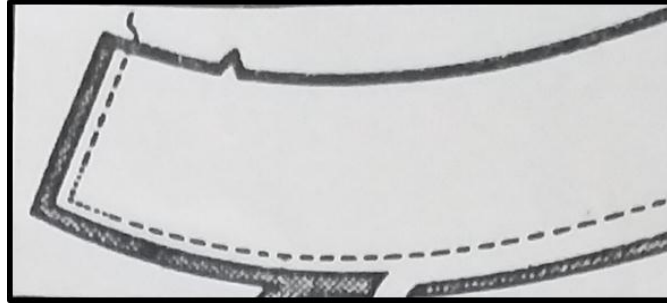
شكل ( ١ ) التدرج بعرض العلاوات لتقليص سمك الخياطات التي تكوى الى جهة واحدة
