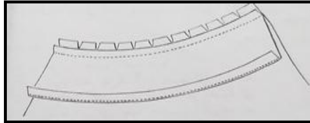
شكل ( ٢ ) تقليص سمك لخياطات المقعرة بقرض العلاوات عرضيا لراحة حافاتها ومنع انكماشها عندما تكوى الى جهة واحدة
