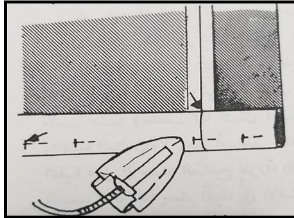
شكل ( ١٦ ) مطابقة الخياطات الطولية وكسر خط الثنية بالمكواة
