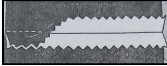
شكل ( ٥ ) قص الحافات بالمقص المسنن
