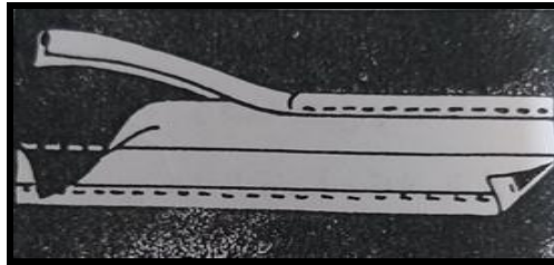
شكل ( ١٠ ) تغطية الحافة السائبة بشريط
